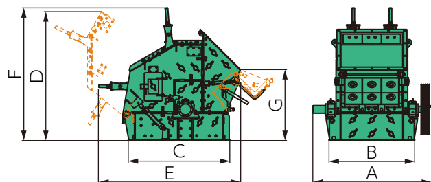
一次破碎機
