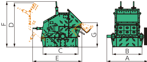
一次破碎機
