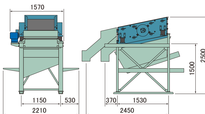
HV35F (電動タイプ)
