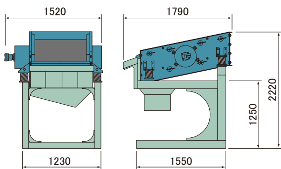
HVVH35E (油圧タイプ)
