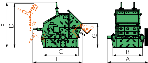
一次破碎機
